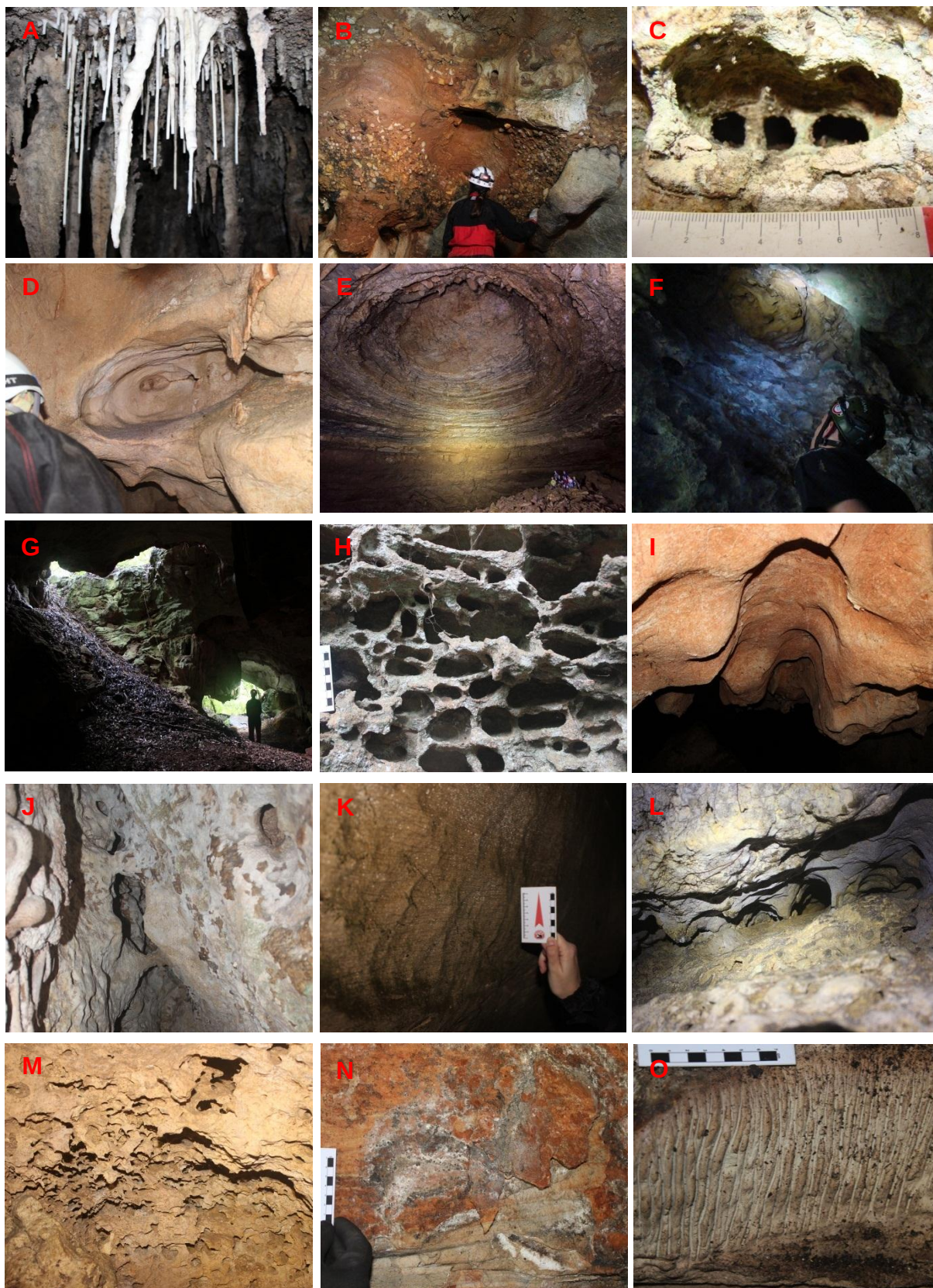
FIGURA 2.2 - FEIÇÕES GEOLÓGICAS DE CAVERNAS: A) ESPELEOTEMAS; B) DEPÓSITOS CLÁSTICOS; C) DUTOS DE DISSOLUÇÃO; D) CÚPULAS DE DISSOLUÇÃO; E) DOMOS; F) CHAMINÉ DE EQUILÍBRIO; G) CLARABOIA; H) ALVÉOLOS; I) CANAIS DE TETO; J) CANAIS DE PAREDE; K) SCALLOPS; L) ALIMENTADORES; M) ANASTOMOSE; N) INCRUSTAÇÃO E; O) SULCOS VERTICAIS (FOTOS: HENRIQUE SIMÃO PONTES; FOTO E: CSX CORPORATION).
