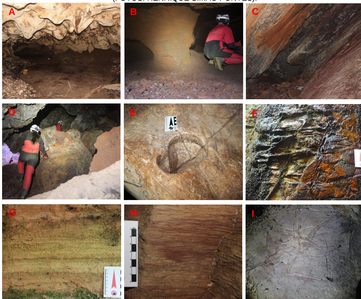
FIGURA 2.3 - FEIÇÕES GEOLÓGICAS DE CAVERNAS: A) PENDENTES; B) PILARES; C) PONTÕES ESTRUTURAIS; D) PATAMARES; E) PANEIS; F) BOXWORKS ; G) ROCHA FANTOMIZADA/ARENIZADA; H) ESTRUTURAS GEOLÓGICAS E; I) ICNOFÓSSEIS (FOTOS: HENRIQUE SIMÃO PONTES).
