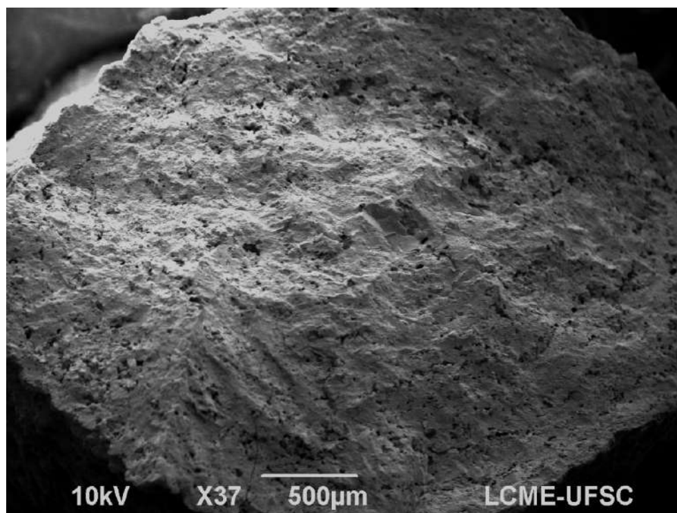
Figura 6.39 – Imagem de MEV de corte transversal na amostra SAC 4. A superfície interna é caracterizada por uma massa amorfa de textura porosa. Nesta seção é possível ver melhor a estrutura em camadas rítmicas concêntricas.
