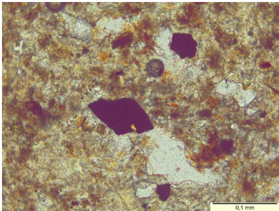
Figura 6.58 – Grãos de magnetita (mineral acessório do Granito Ilha) na matriz amorfa do espeleotema cilíndrico de piso (amostra SAC 4) a nicóis paralelos.
