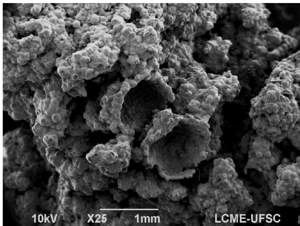
Figura 6.41 – Imagem de MEV da superfície externa de coraloide arborescente (amostra GSG 1A). A textura é globular, formada por microesferas colmatadas.
