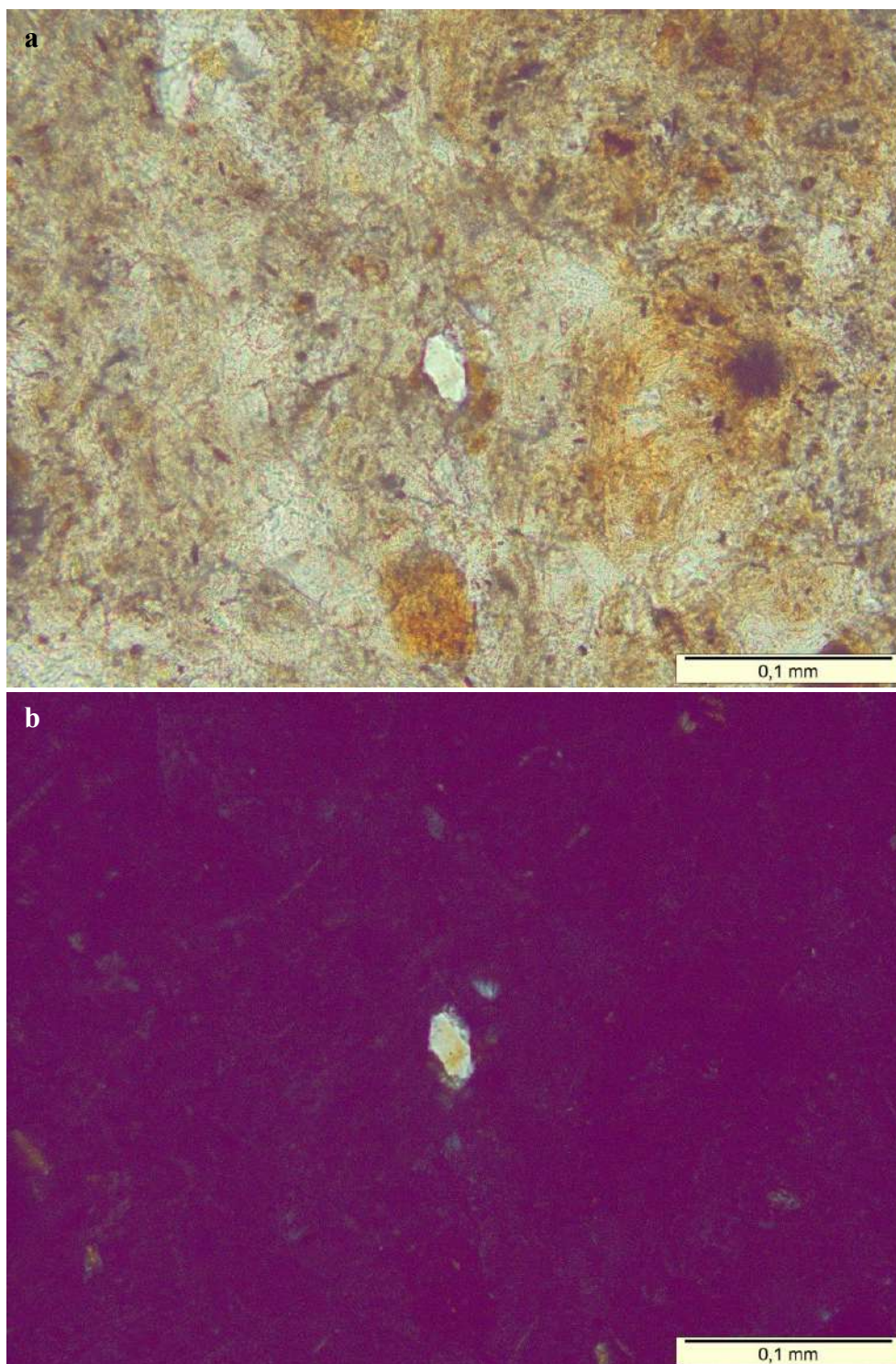
Figura 6.55 – Grão de quartzo na matriz amorfa do espeleotema cilíndrico de teto (amostra SAC 5A): a) imagem com nicóis paralelos; b) imagem com nicóis cruzados.
