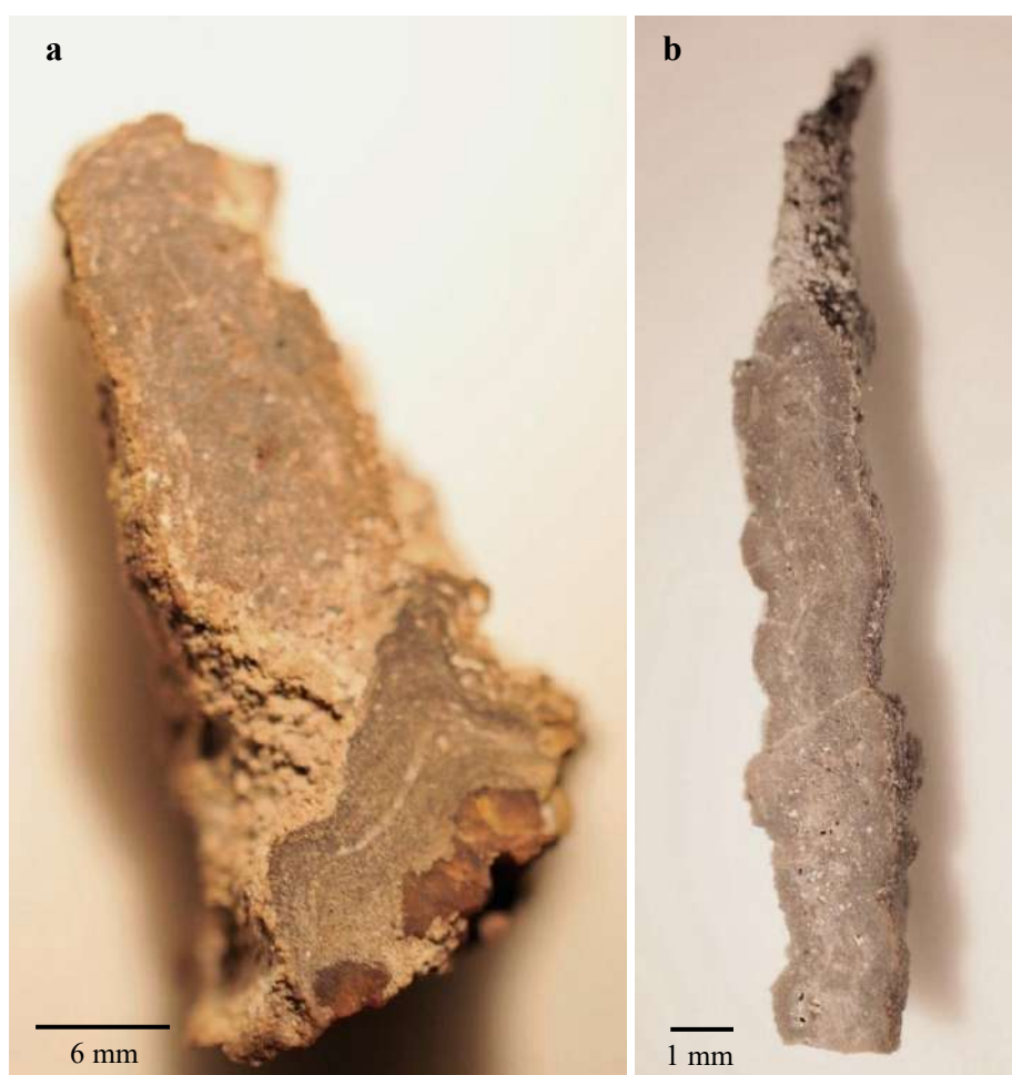
Figura 6.47 – Cortes longitudinais nos espeleotemas cilíndricos: a) amostra SAC 4 evidenciando a estrutura organizada em camadas rítmicas, especialmente na porção basal; b) amostra SAC 5A ( porção intermediária e apical) onde é nítida a estrutura organizada em camadas rítmicas a partir de um eixo de crescimento também longitudinal.
