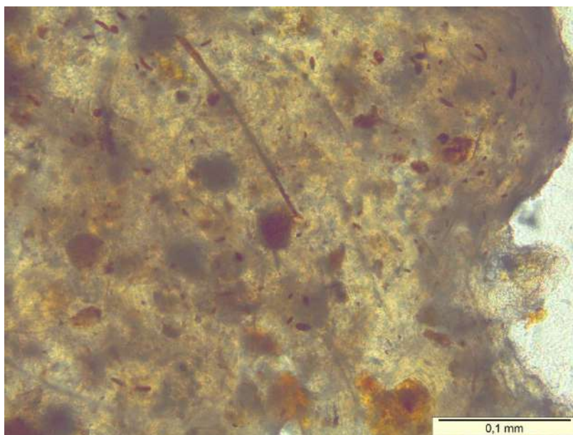
Figura 6.54 – Setor apical da amostra SAC 5A ao microscópio ótico (nicóis paralelos). A matriz tem coloração clara e aspecto fosco/enevado. Os elementos arredondados e aciculares representam grãos de minerais detríticos e material biológico.
