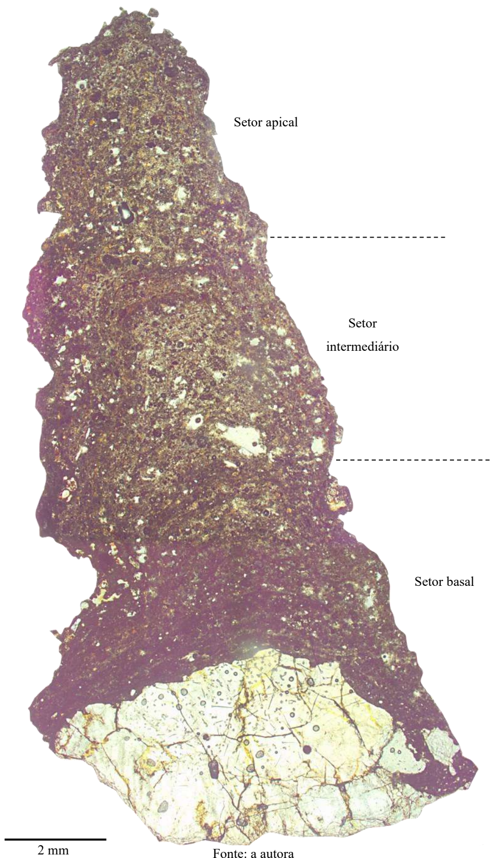
Figura 6.48 – Lâmina da amostra SAC 4 (nicóis paralelos), dividida em setores a partir de suas características estruturais. Espeleotema assentado sobre o substrato granítico (aqui, apenas cristais de quartzo).
