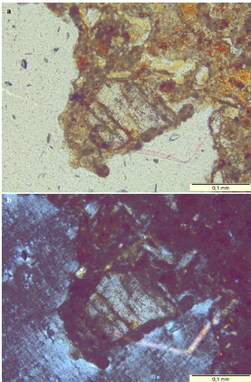
Figura 6.56 – Grão de feldspato na matriz amorfa do espeleotema cilíndrico de piso (amostra SAC 4): a) imagem com nicóis paralelos; b) imagem com nicóis cruzados.
