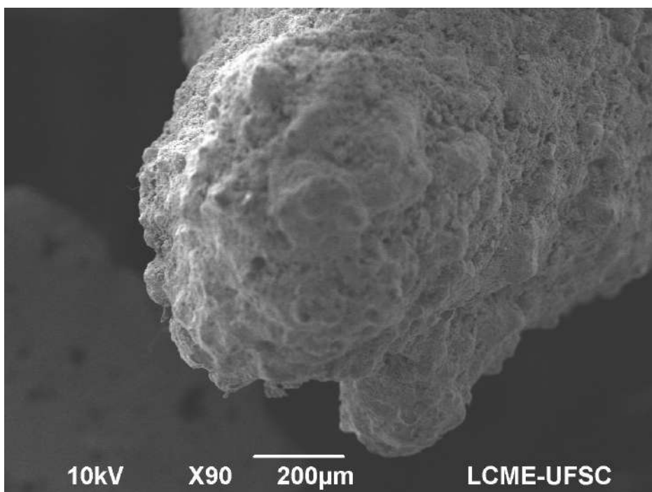
Figura 6.36 – Imagem de MEV da ponta da amostra SAC 5A, apresentando uma superfície irregular, de aspecto rugoso-granular.
