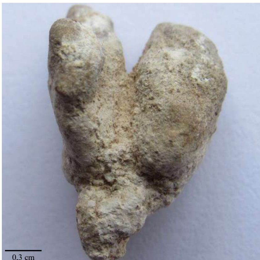
Figura 6.51 – Aspectos da morfologia do coraloide nodular (amostra SAC 12).
