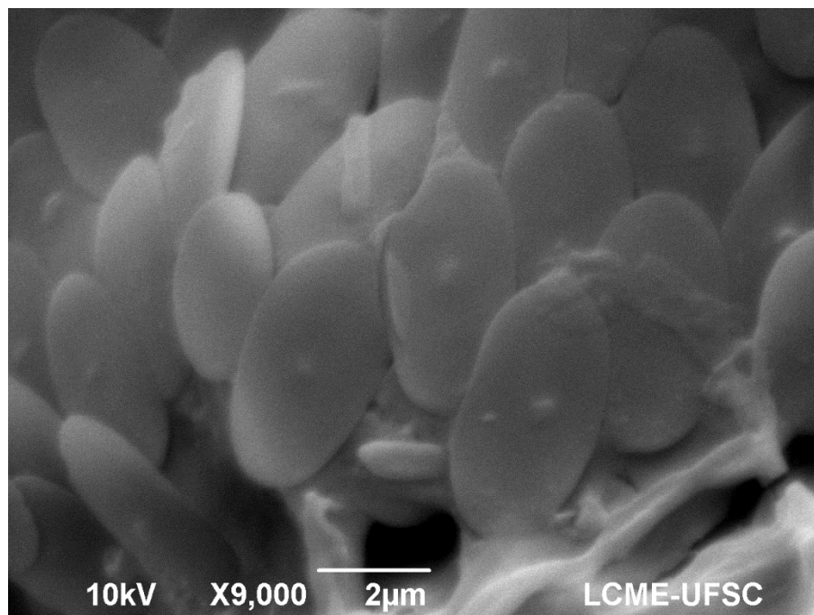
Figura 6.71 – Detalhe das escamas de sílica que dão corpo à teca da Figura 6.70b. O gráfico da análise de EDS de uma das escamas mostra a participação predominante do Si (40,64%) C (31,69%) e O (19,49%), seguidos de N (7,12%) e Al (1,06%). O pico sem identificação é do ouro utilizado no recobrimento da amostra.
