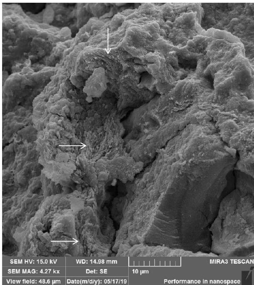
Figura 6.63 – Aspecto laminar/foliado de um setor do flowstone (amostra SAC 14), característica da birnessita. Um indício de que este pode ser o mineral de óxido de manganês que compõe o espeleotema.
