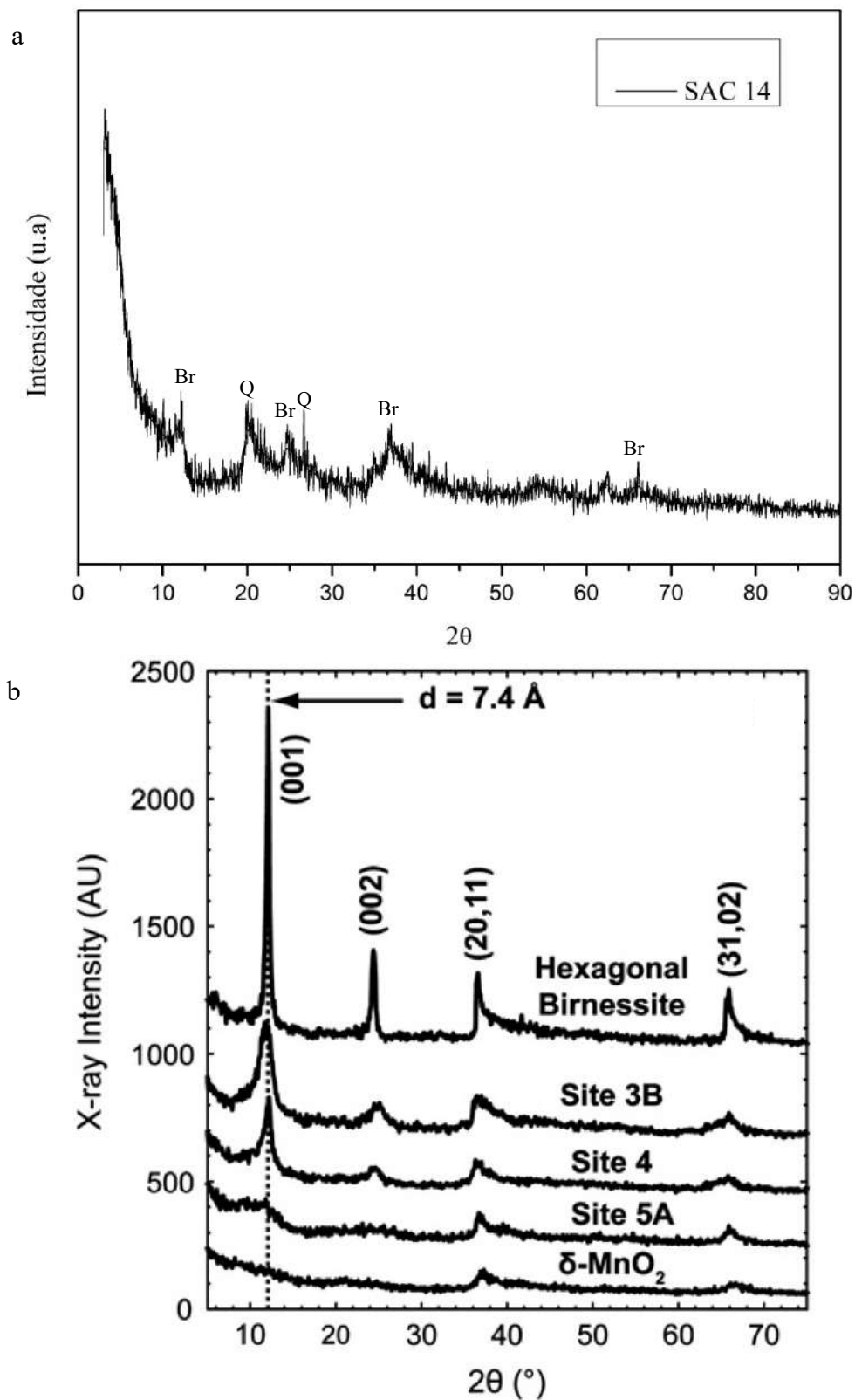
Figura 6.62 – Difratomogramas da amostra SAC 14 e de materiais compostos por birnessita, para comparação: a) amostra do flowstone coletado no SAC com indicação das prováveis fases cristalinas, por comparação (Br – birnessita; Q – quartzo- \alpha ); b) amostras de depósitos de óxido de manganês da Pautler Cave, sudoeste de Illinois (EUA).
