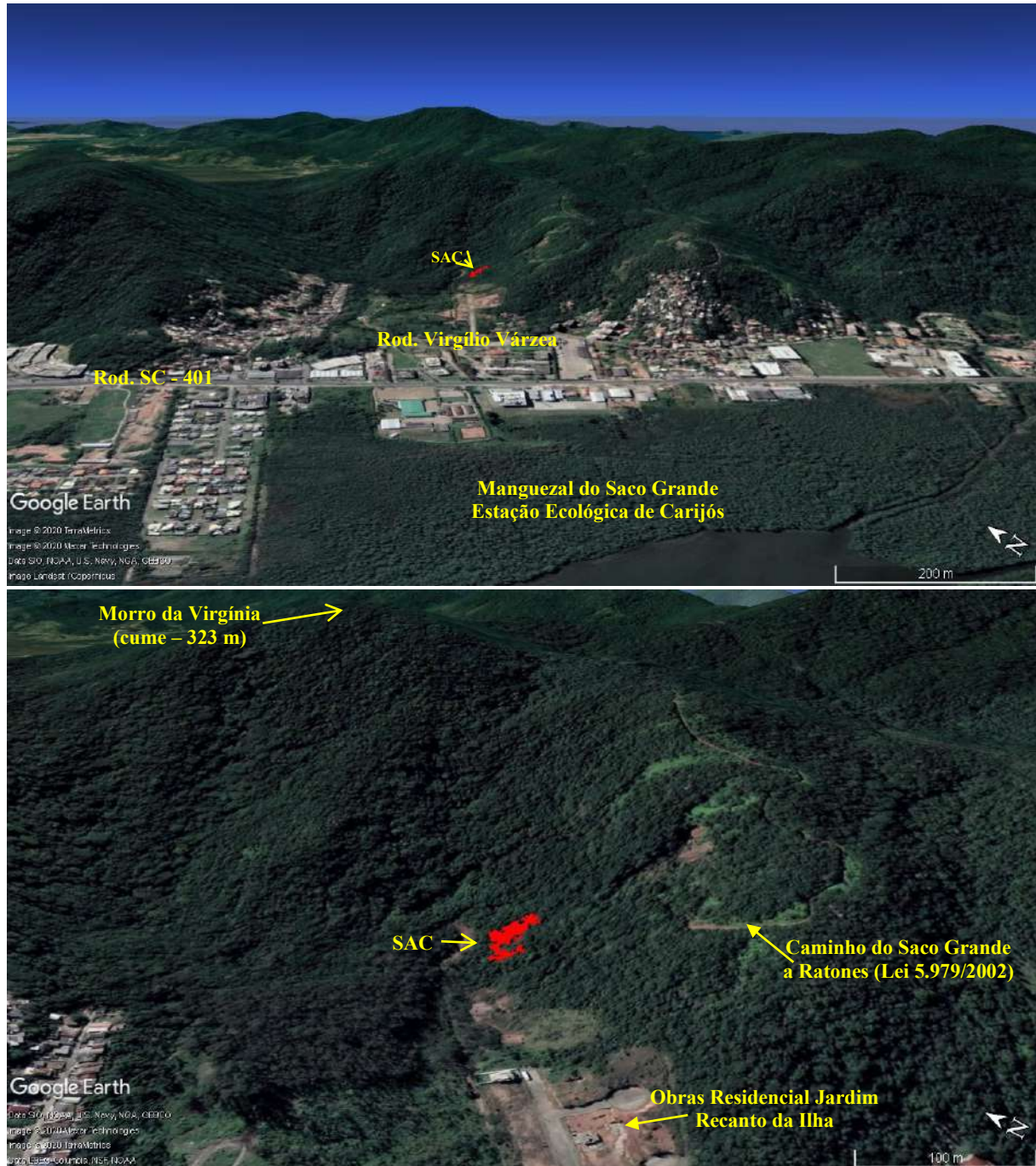
Figura 5.5 – Imagens de satélite em perspectiva 3D da área onde está situado o SAC.
