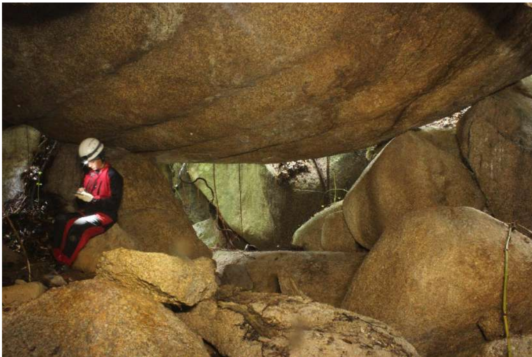
Figura 5.47 – Caneluras com relevo suave dispostas na horizontal em matacão que compõe o teto da caverna.
