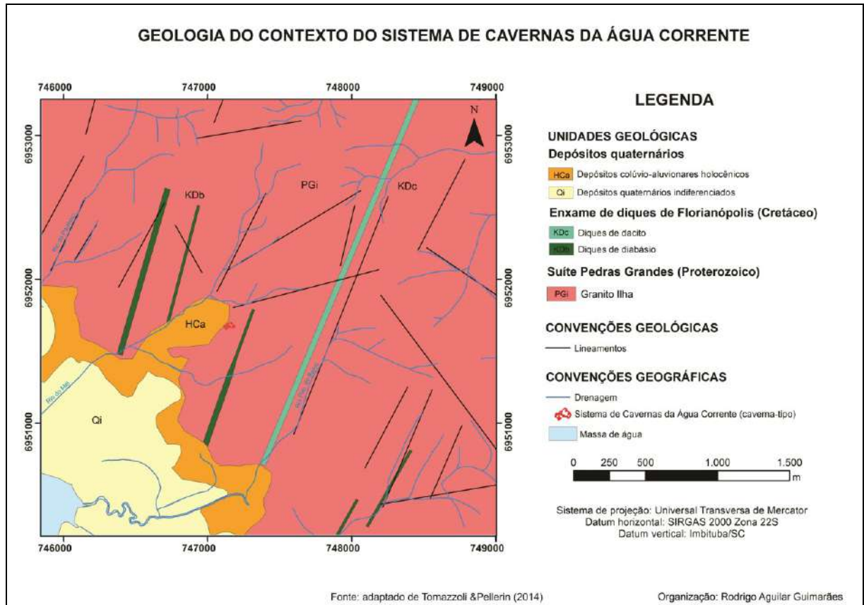
Figura 5.1 – Contexto geológico do Sistema de Cavernas da Água Corrente.
