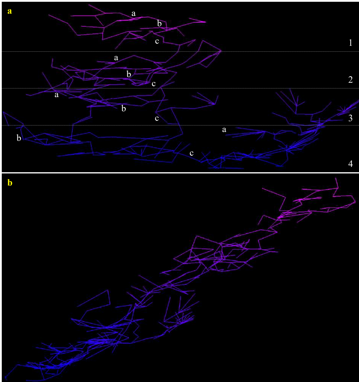
Figura 5.6 – Modelos tridimensionais do SAC extraídos do aplicativo TopoDroid : a) seção WSW/ENE com a identificação dos 4 níveis principais e subníveis; b) projeção vertical da seção descrita em “a”.
