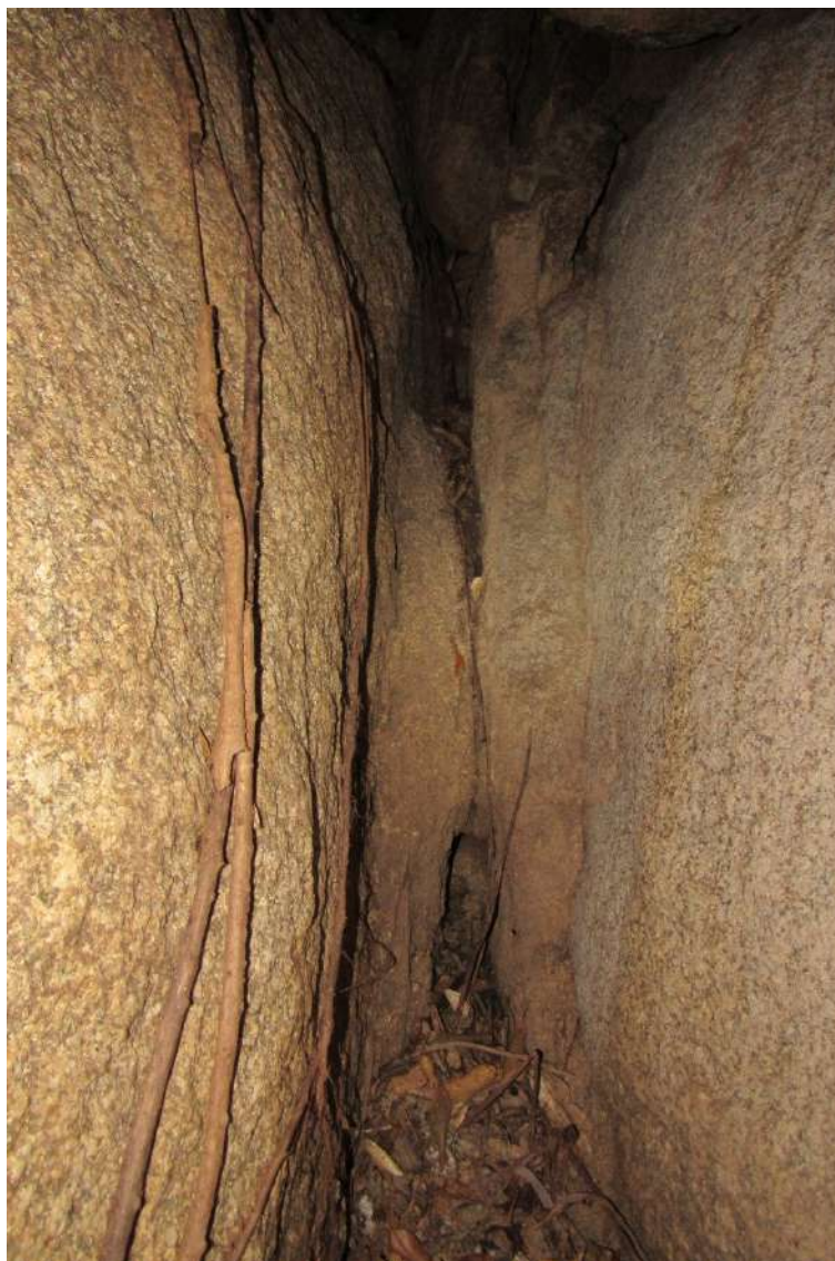
Figura 5.36 – Matacões parcialmente expostos formando a parede de uma galeria do SAC. Entre ambos é possível ver a descamação esferoidal e a ação do intemperismo individualizando as massas rochosas.
