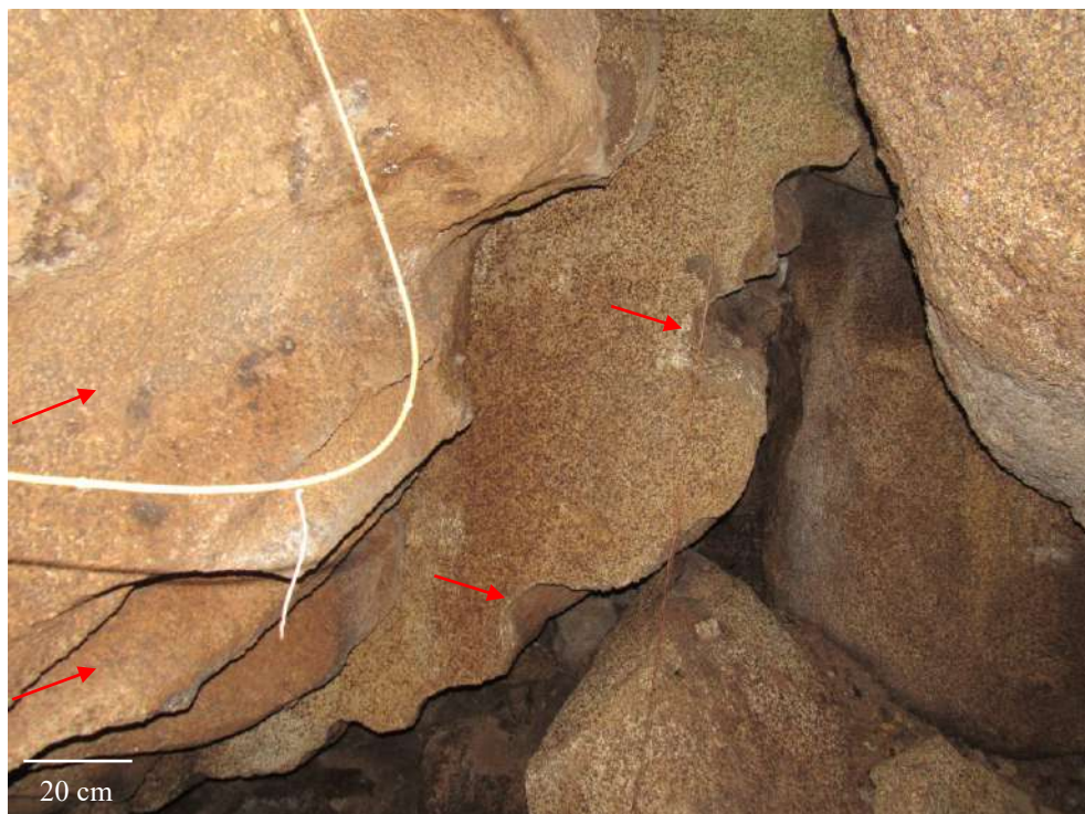
Figura 5.71 – Matacões com caneluras dispostas na posição horizontal (ver setas) evidenciando o movimento e rotação dos mesmos – Gruta do Oiteiro.
