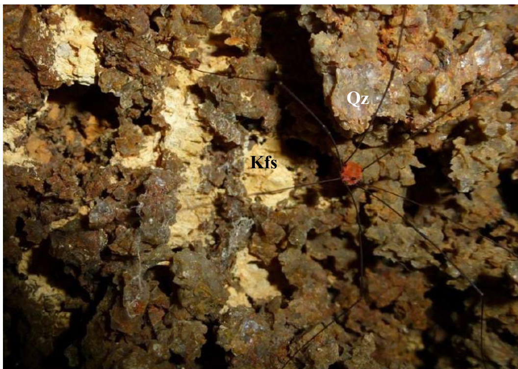
Figura 6.82 – Contraste entre o quartzo (Qz), em relevo e desprovido de sinais de alteração, e o feldspato potássico (Kfs), já alterado para caulinita – Gruta do Riacho Subterrâneo. O opilião tem um corpo (cefalotórax + abdômen) de ~3 mm.
