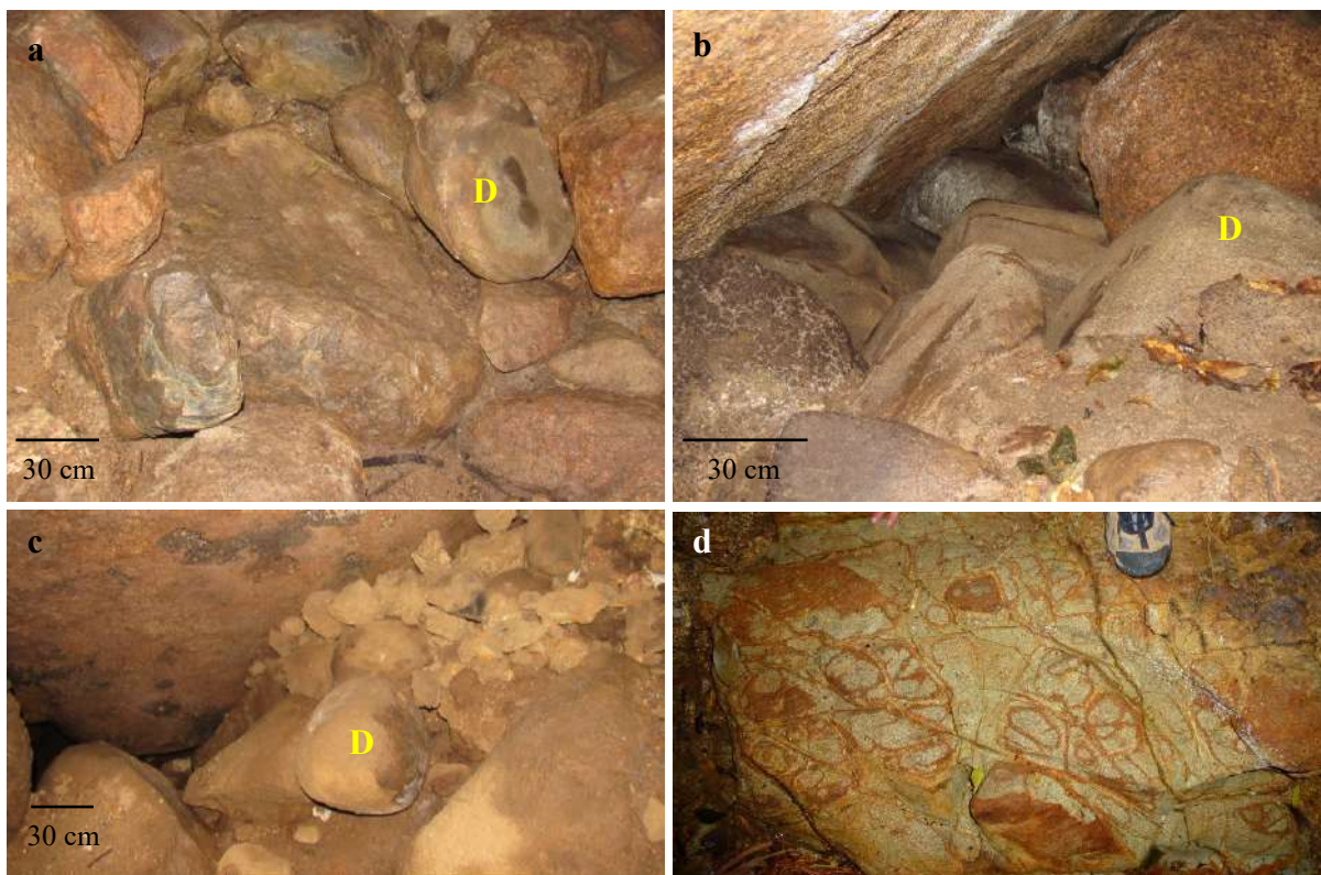
Figura 5.66 – Presença do diabásio (D) em outras cavernas em matacões graníticos da ISC: a e b) matacões e blocos em diferentes compartimentos da Gruta das Feiticeiras; c) pequenos matacões esféricos na Gruta do Oiteiro; d) dique na Gruta da Jararaca.
