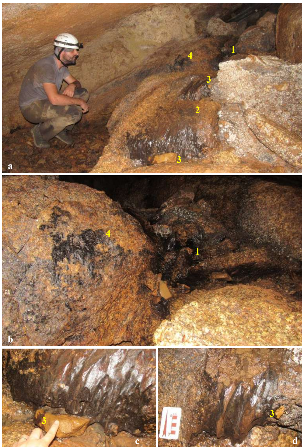
Figura 6.33 – Ocorrência de flowstone no leito (1) e nas margens (2) de um pequeno curso d'água que corta o SAC. O material precipitado envolve seixos associados à drenagem e ruditos (3) e em alguns locais aparece polido (3) e desgastado pela erosão fluvial (4). As imagens b, c e d são detalhes de setores em a.
