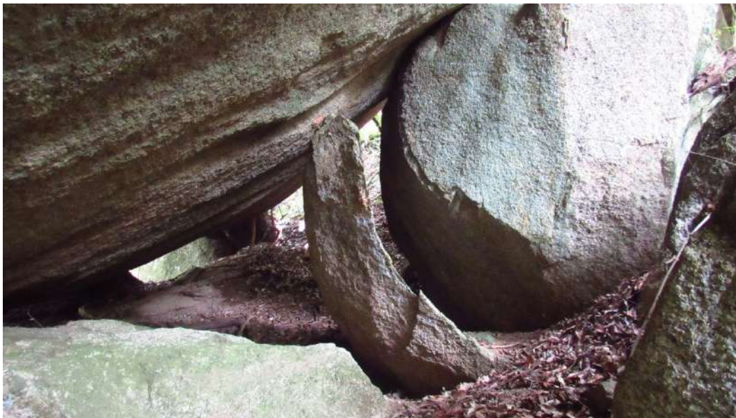
Figura 5.37 – Grande fragmento de contornos curvilíneos, indicando a atuação de descamação esferoidal, destacado do matacão original à sua direita.
