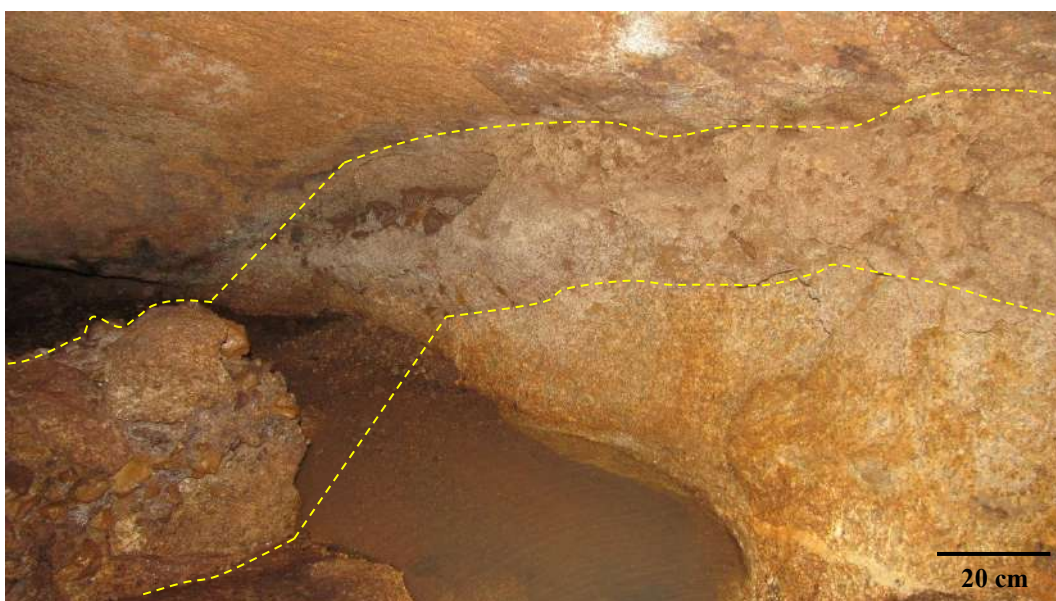
Figura 5.43 – Descontinuidade da camada conglomerática mais expressiva do SAC, erodida por ação fluvial. Do lado direito da drenagem porções residuais estão dispostas junto à parede, enquanto na margem esquerda há disposição descontínua, no piso ao longo de toda a galeria.
