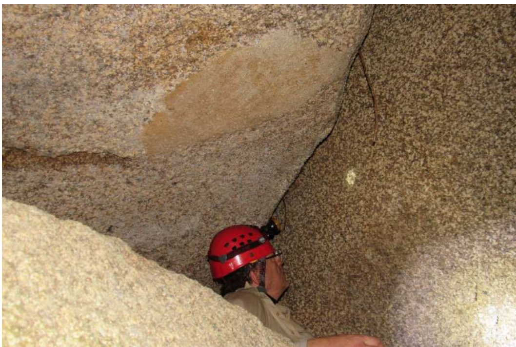
Figura 5.26 – Enclave microgranular leucocrático (composição ácida) com formato elipsoidal e cerca de 60 cm de diâmetro (mancha em evidência acima da cabeça do espeleólogo).
