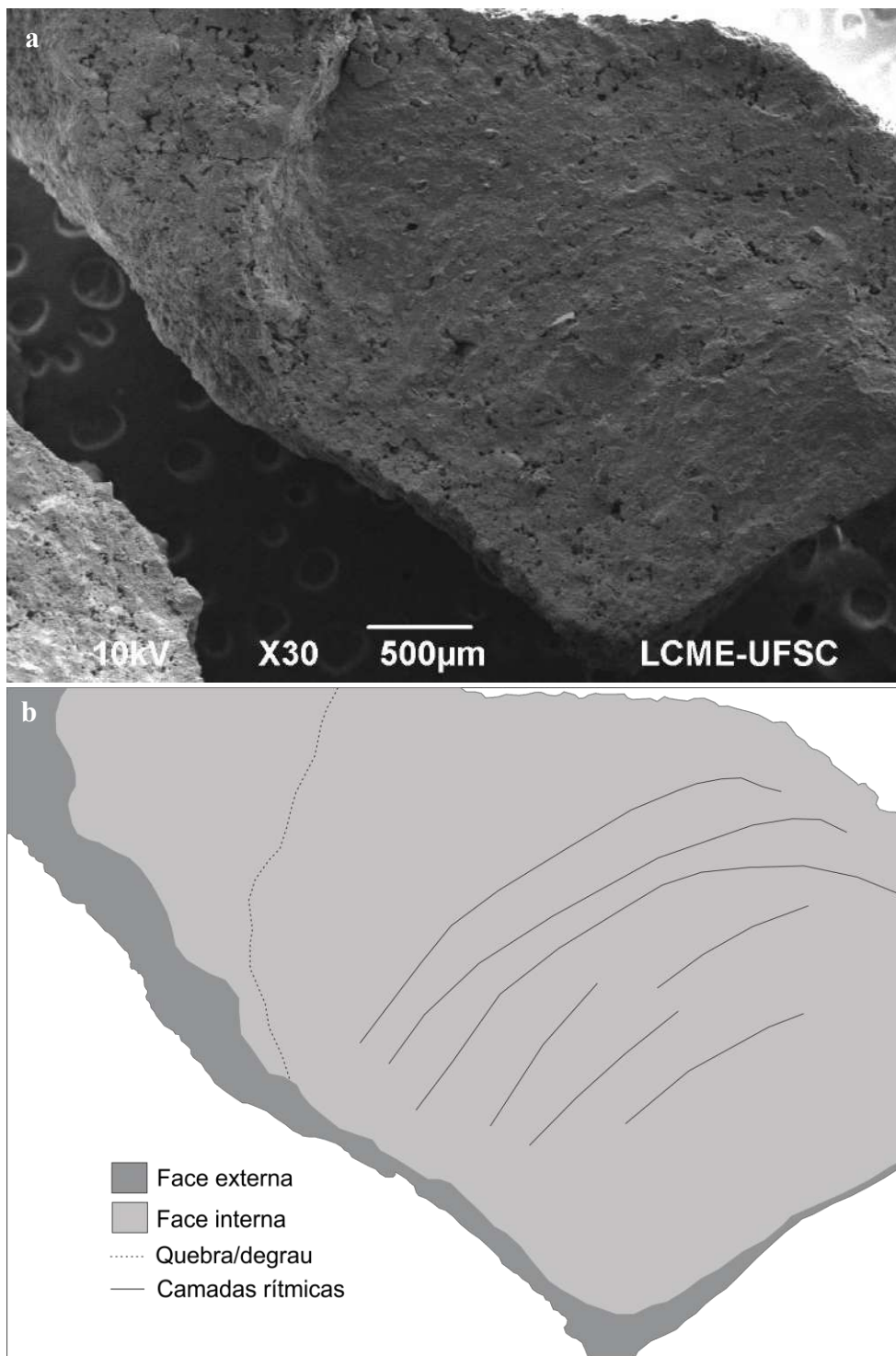
Figura 6.37 – Corte longitudinal da amostra SAC 4: a) a superfície externa é irregular, de textura rugosa, já a face interna mostra que a massa amorfa tem aspecto poroso; b) croqui da Figura 6.37a, evidenciando a estrutura interna organizada em camadas rítmicas, sutil na imagem de MEV.
