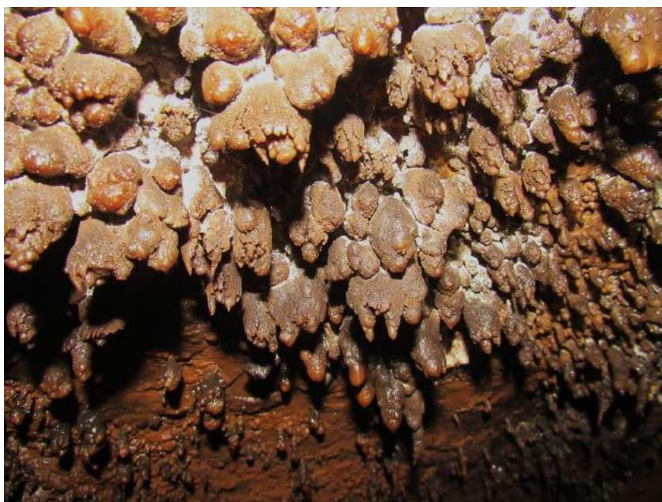
Figura 6.14 – Detalhe do conjunto da Figura 6.12. A acreção sucessiva de material recobriu e uniu feições antes individualizadas, formando um núcleo de espeleotemas mais desenvolvidos, principalmente em largura.
