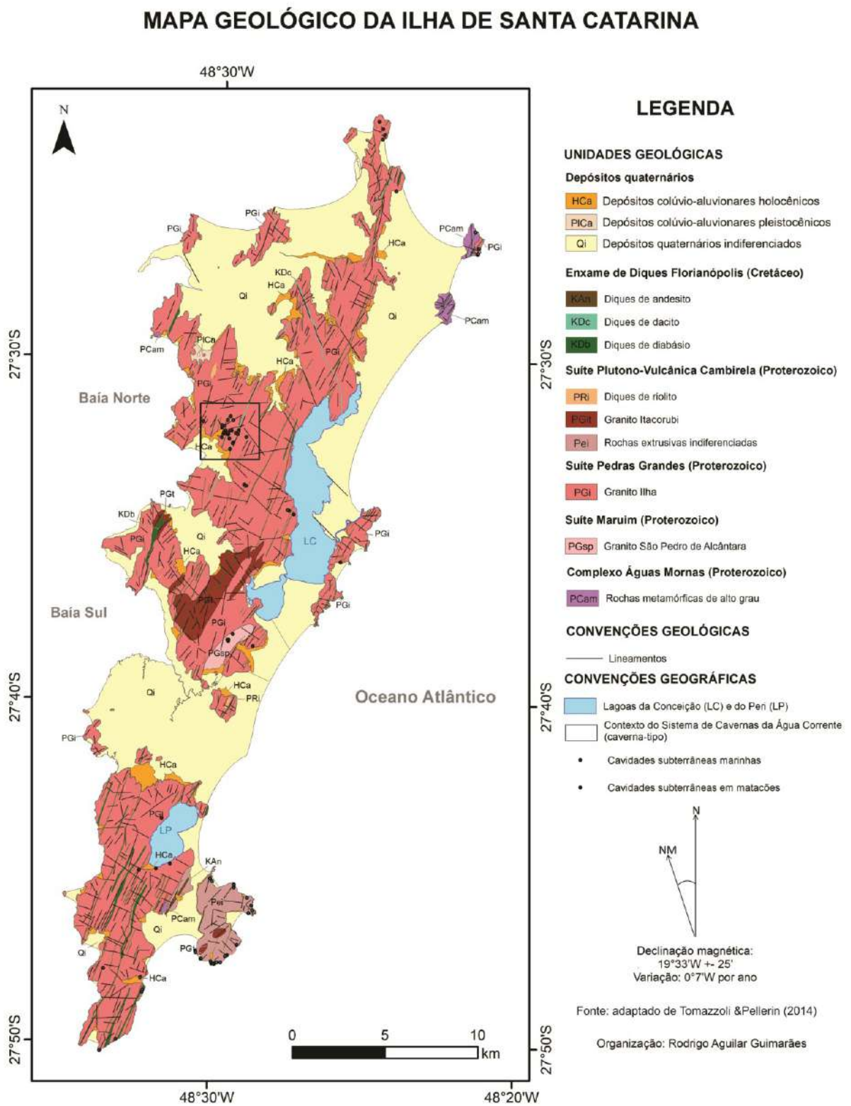
Figura 2.2 – Geologia da Ilha de Santa Catarina com a localização das cavidades subterrâneas em matacões e marinhas e indicação do contexto do Sistema de Cavernas da Água Corrente.
