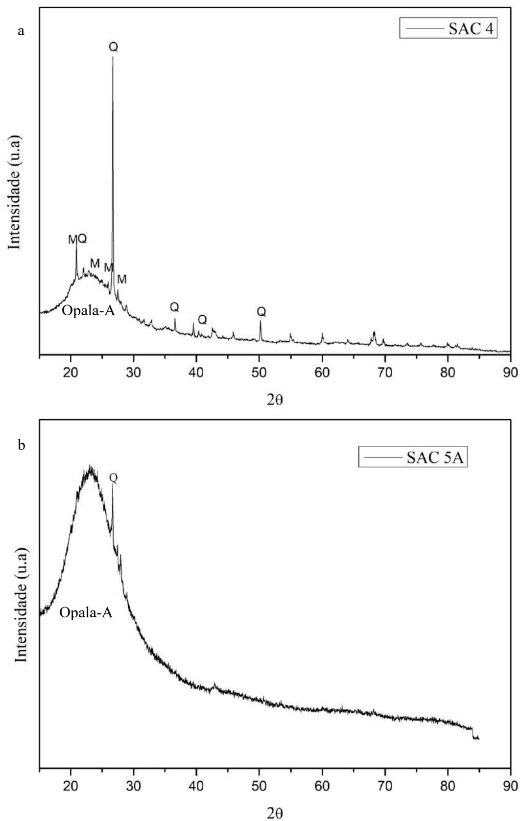
Figura 6.59 – Difratomogramas dos espeleotemas cilíndricos: a) SAC 4 (piso); b) SAC 5A (teto) (Q = quartzo- \alpha ; M = microclínio).
