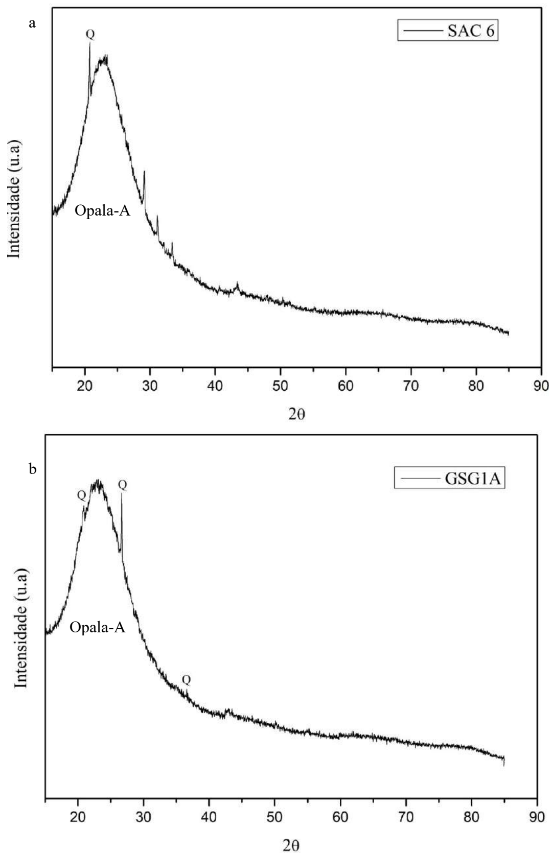
Figura 6.60 – Difratomogramas dos espeleotemas coraloídes arborescentes: a) SAC 6; b) GSG 1A (Q = quartzo- \alpha ).
