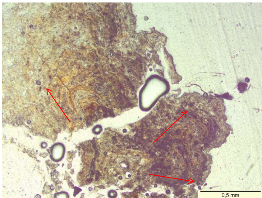
Figura 6.50 – Lâmina de um fragmento da amostra SAC 6 (nicóis paralelos). As camadas rítmicas acompanham as ramificações do espeleotema (setas). As bolhas e fraturas representam defeitos na confecção da lâmina, em função da porosidade e fragilidade do material.
