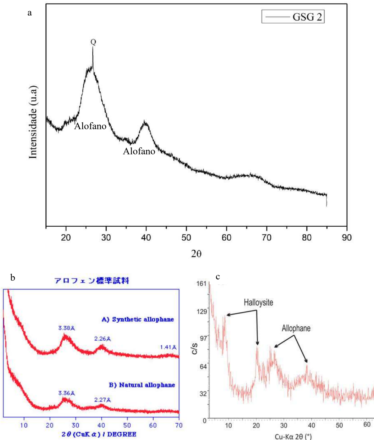
Figura 6.64 – Difratomogramas da amostra GSG 2 e de materiais compostos por alofano, para comparação: a) amostra do flowstone coletado na Gruta do Saco Grande (Q = quartzo- \alpha ); b) amostras de alofano sintético e natural, figura obtida em um banco de difratogramas; c) amostra de espeleotema associado a raízes proveniente de uma caverna vulcânica (Açores).
