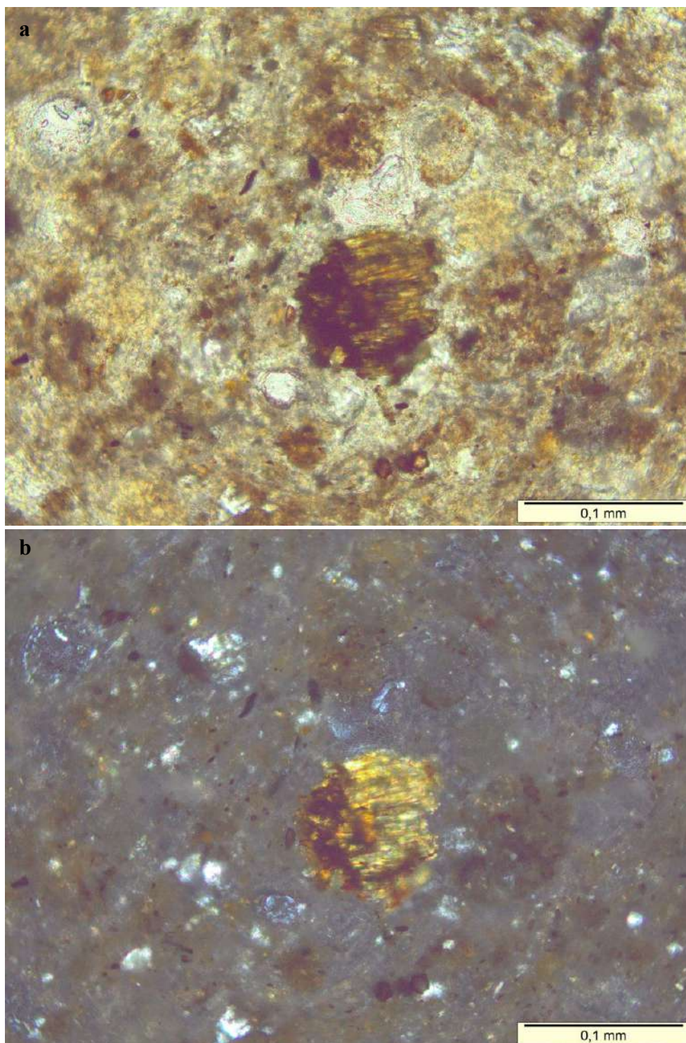
Figura 6.57 – Grão de biotita na matriz amorfa do espeleotema cilíndrico de piso (amostra SAC 4): a) imagem com nicóis paralelos; b) imagem com nicóis cruzados.
