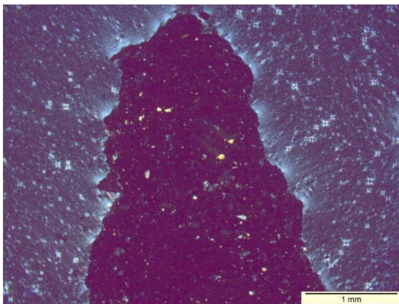
Figura 6.53 – Setor apical e parte do setor intermediário da amostra SAC 4 ao microscópio ótico (nicóis cruzados). A matriz amorfa é isótropa, já os pequenos pontos com birrefringência são grãos detríticos de minerais como quartzo, feldspato e biotita.
