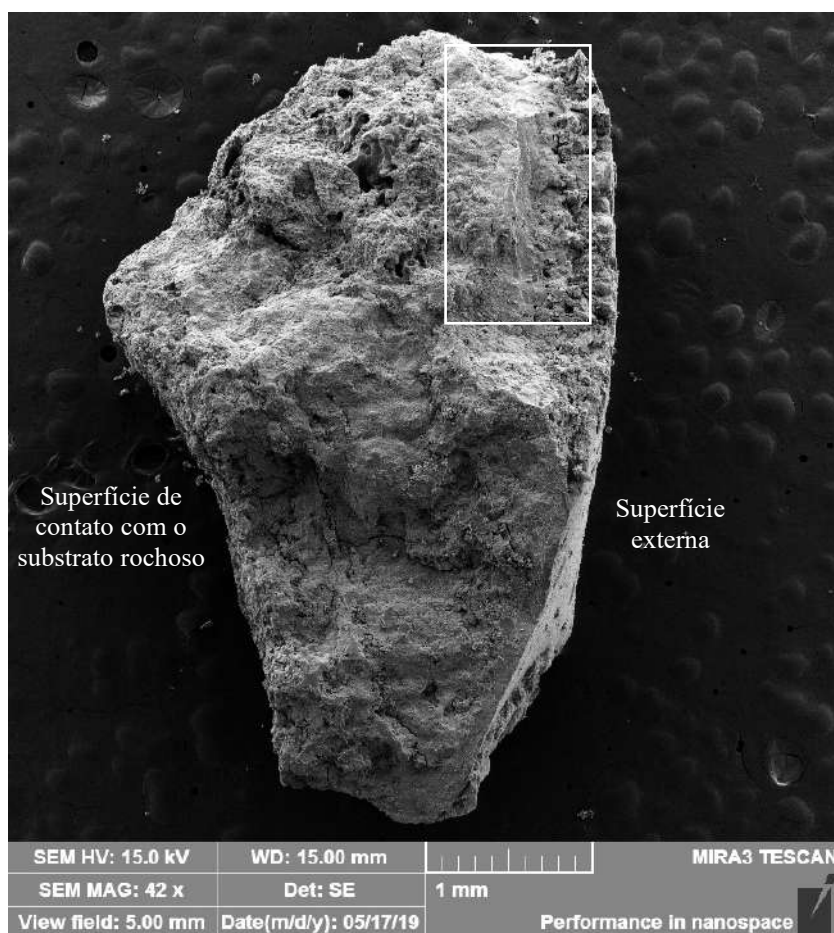
Figura 6.44 – Imagem de MEV do perfil da crosta que constitui o flowstone (amostra SAC 14). Em destaque, setor com estrutura estratificada.
