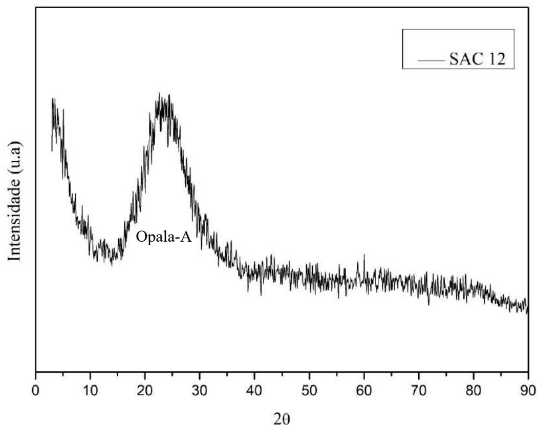
Figura 6.61– Difratoograma do espeleotema coraloide nodular – SAC 12.
