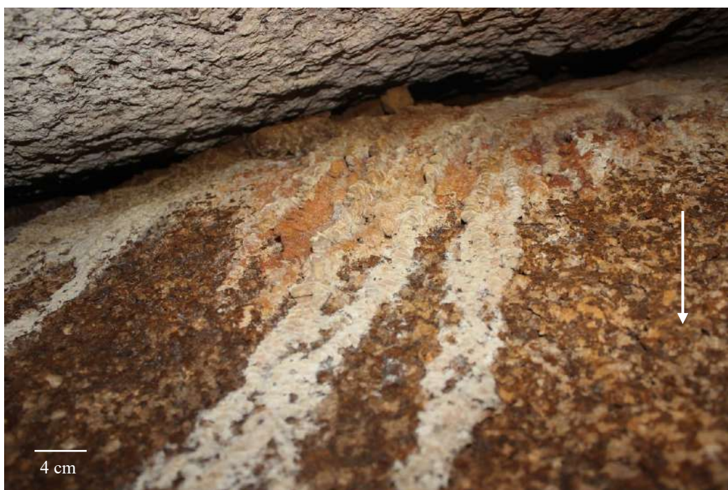
Figura 6.35 – Flowstone associado à circulação concentrada da água (a seta indica o sentido do fluxo) em pontos próximos, gerando feições lineares paralelas em parede na Gruta do Saco Grande (local de coleta da amostra GSG 2, submetida às análises de MEV e DRX).
