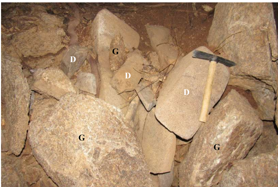
Figura 5.38 – Depósito clástico gravitacional no piso do SAC formado por matacões, blocos e seixos de granito (G) e diabásio (D). Depósitos similares em outros pontos da caverna também incluem fragmentos de duricrust ferruginoso.
