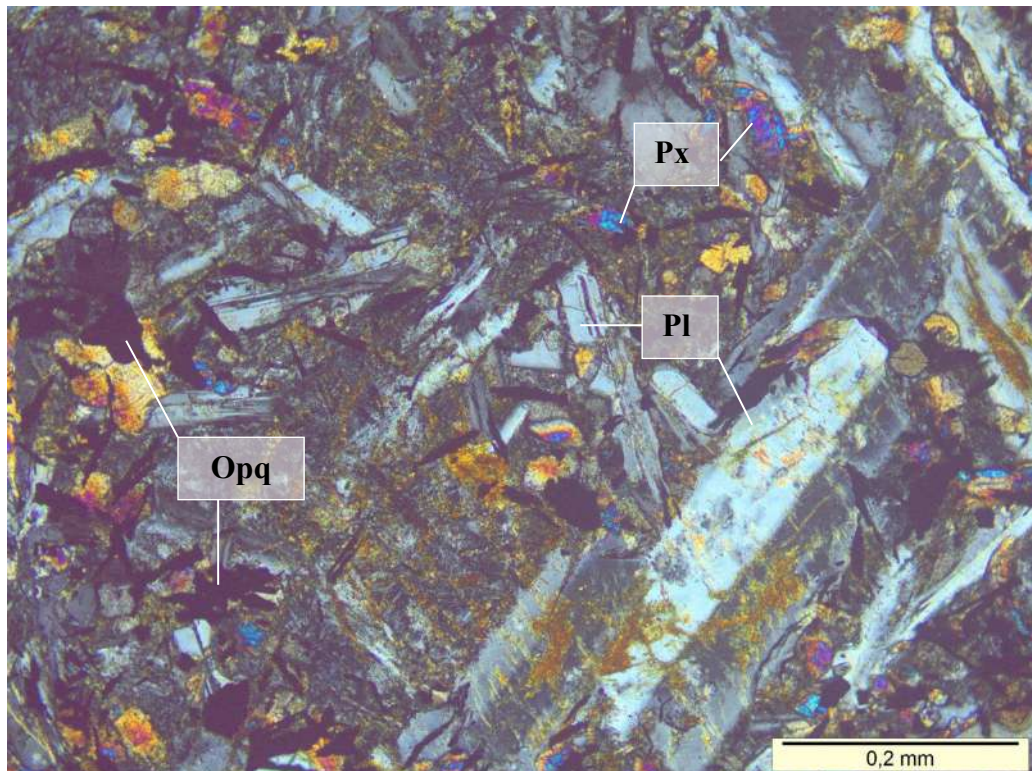
Figura 5.23 – Lâmina delgada da amostra SAC 9 (nicóis cruzados) mostrando seus minerais primários (Pl – feldspato plagioclásio; Px – piroxênios; Opq – minerais opacos).
