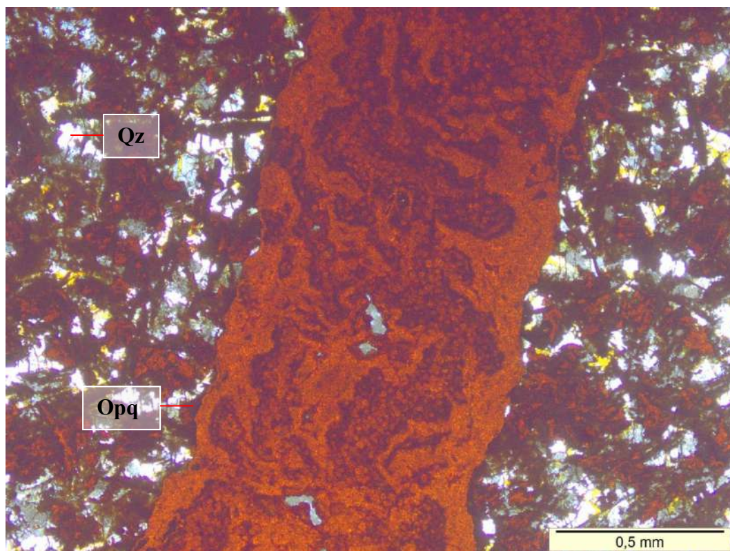
Figura 5.40 – Lâmina delgada da amostra SAC 10 mostrando grãos de quartzo (Qz), minerais opacos (Opq) e uma faixa com maior concentração de hidróxido de ferro.
