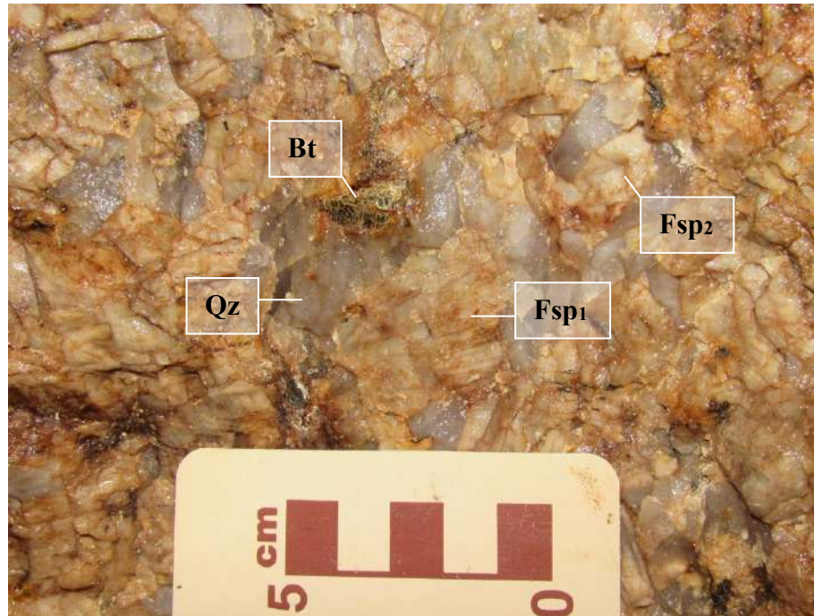
Figura 5.33 – Veio (ou bolsão) pegmatítico com os mesmos minerais primários do granito, porém com dimensões maiores (Qz – quartzo; Bt – biotita; Fsp 1 – feldspato potássico; Fsp 2 – feldspato plagioclásio [?]).
