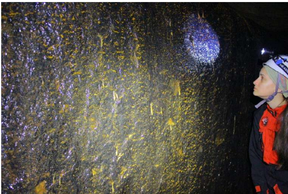
Figura 6.30 – Aproximação no espeleotema da Figura 6.29. A água escorre de forma lenta, como um lençol sobre a rocha.
