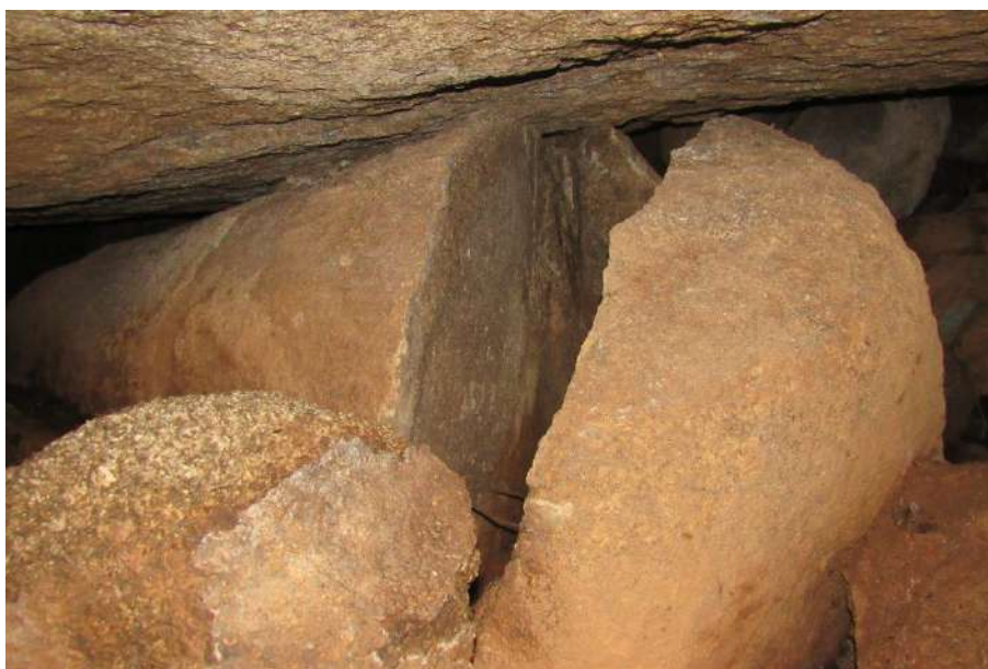
Figura 5.30 – Dois matacões resultantes da divisão de uma massa maior pela presença e evolução de uma descontinuidade na rocha. A pressão exercida pelo matacão do teto pode ter influenciado na ruptura. Do topo à base da imagem, aproximadamente 1,5 m.
