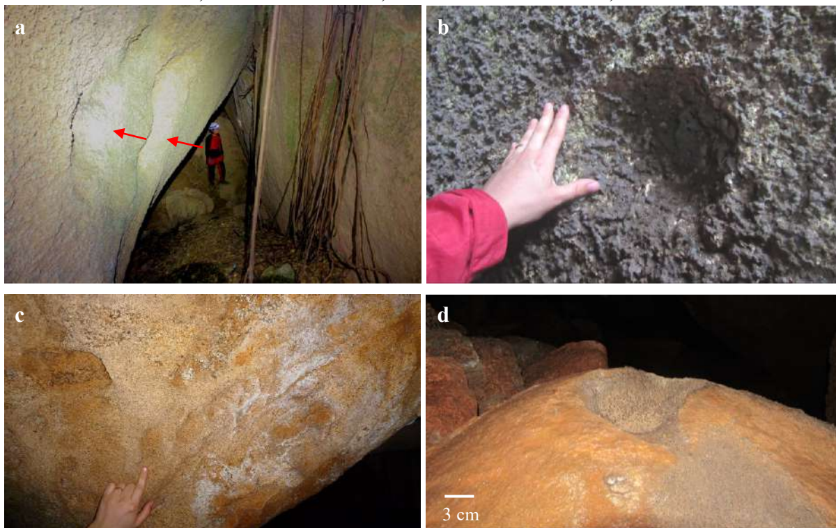
Figura 5.75 – Formas alveolares em outras cavernas em matacões graníticos da ISC: a) Gruta do Saco Grande; b) Gruta do Oiteiro; c) Caverna Central Park; d) Gruta das Feiticeiras.
