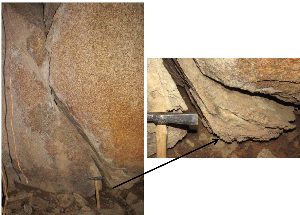
Figura 5.28 – Fratura com segmentos nas posições oblíqua e vertical dividindo um matacão em duas partes. Nas bordas da descontinuidade é possível observar manchas de coloração esbranquiçada relacionadas à alteração da rocha e precipitação de opala, inclusive com a formação de pequenos espeleotemas (ver área próxima à ponta da seta).
