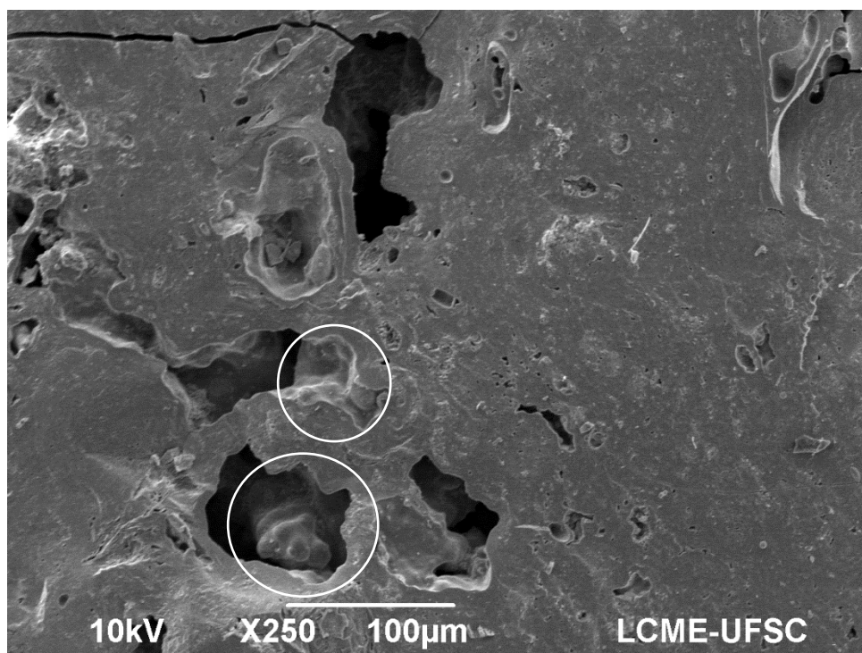
Figura 6.87 – Aspecto textural interno do espeleotema cilíndrico de teto (amostra SAC 5A). Nas poucas áreas porosas é possível ver as microesferas de opala bem coalescidas em função dos processos de redissolução e reprecipitação da opala, que tornam a textura mais compacta e maciça.
