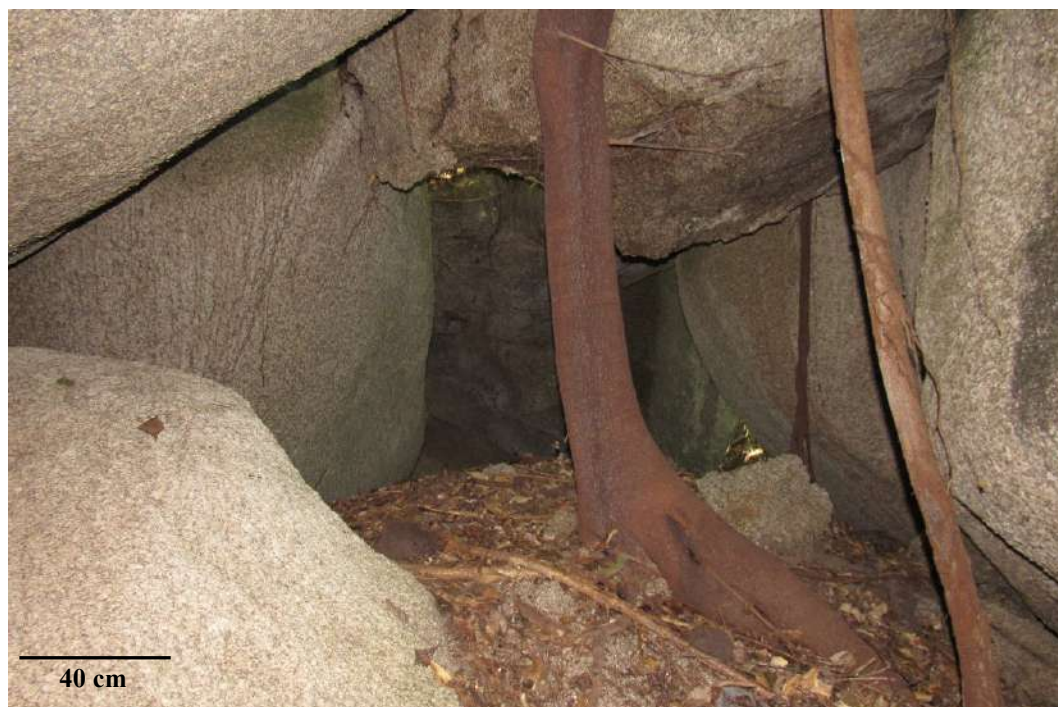
Figura 5.60 – Raízes de árvores adentrando à caverna por aberturas no teto.
