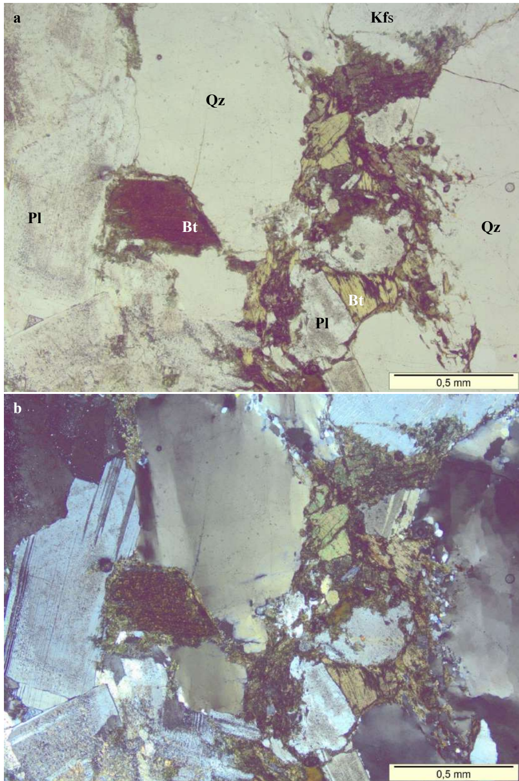
Figura 5.17 – Lâmina delgada da amostra SAC 7 mostrando seus minerais primários (Qz – quartzo; Kfs – feldspato potássico; Pl – plagioclásio; Bt – biotita): a) nicóis paralelos; b) nicóis cruzados.
