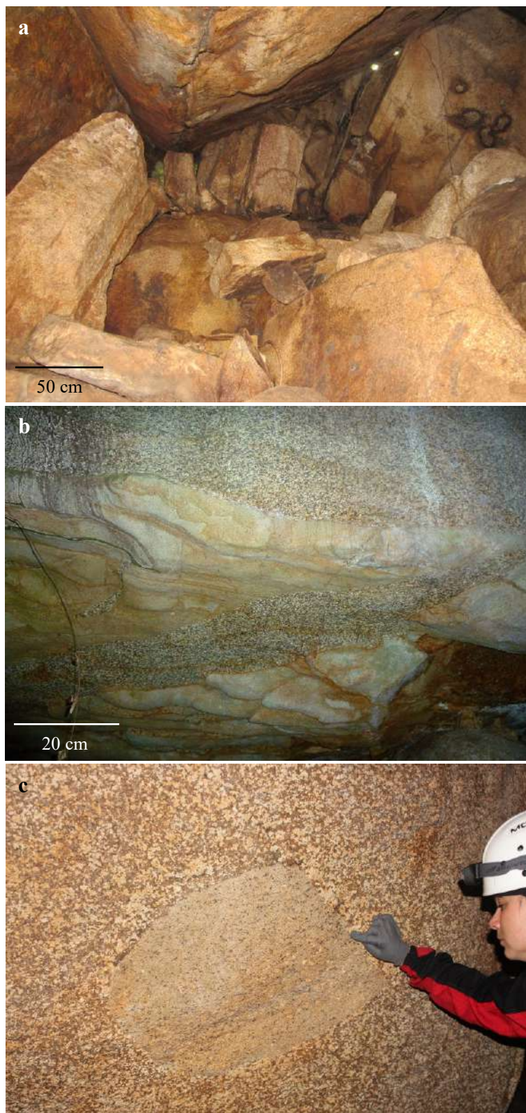
Figura 5.67 – Estruturas tectônicas e ígneas observadas em outras cavernas em matacões graníticos da ISC: a) matacões fraturados na Gruta da Trilha do Saquinho I; b) veio aplítico no teto na Gruta do Saco Grande; c) enclave de composição provavelmente ácida (riolito ?) na Gruta do Saco Grande.
