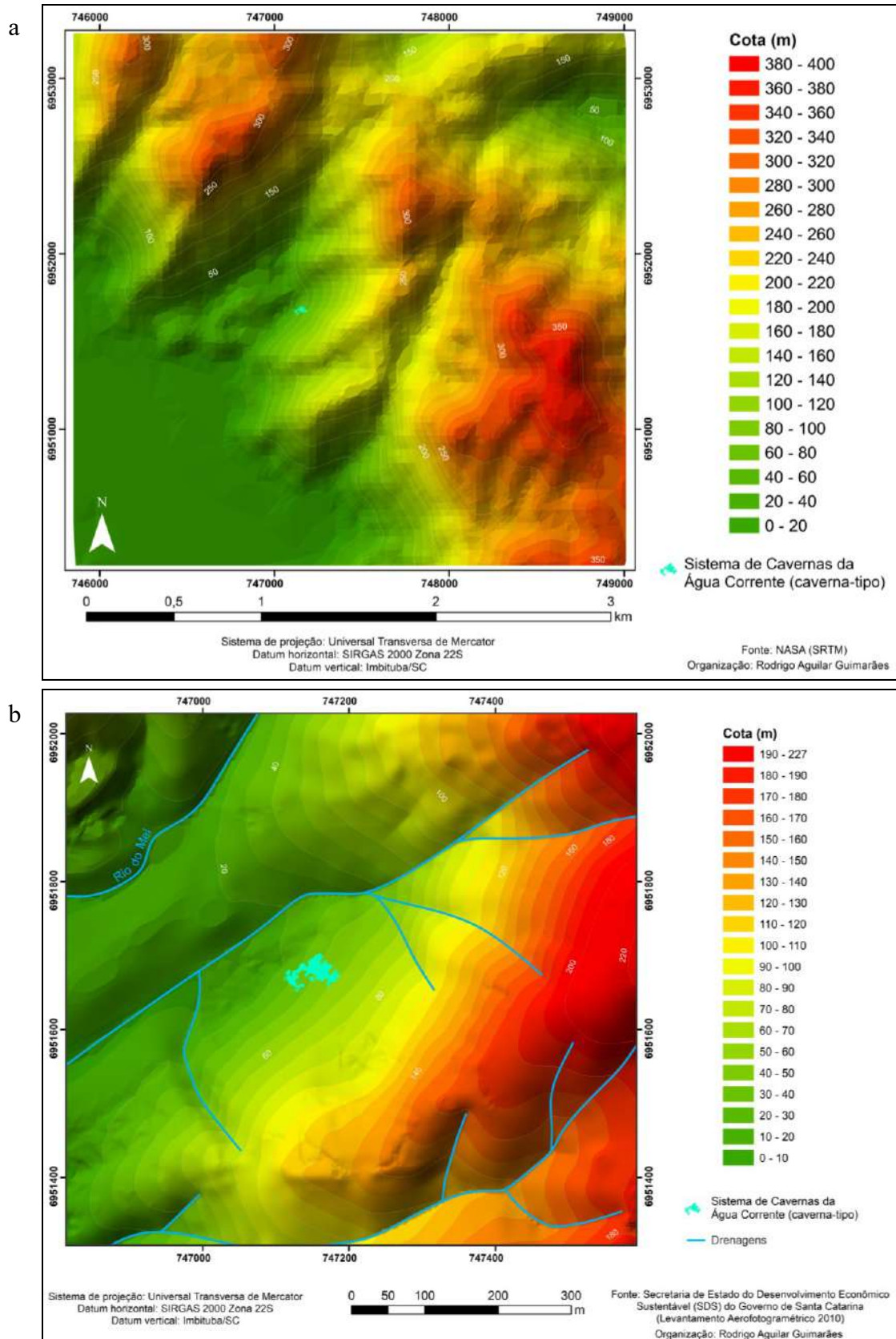
Figura 5.4 – Modelos digitais de elevação do contexto do Sistema de Cavernas da Água Corrente: a) entorno mais amplo; b) entorno imediato.
