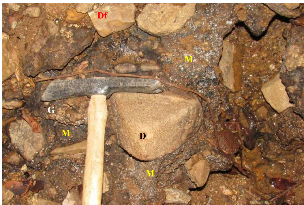
Figura 5.41 – Conglomerado polimítico cimentado por óxidos e hidróxidos de ferro (G – granito; D – diabásio; Df – duricrust ferruginoso; M - matriz).
