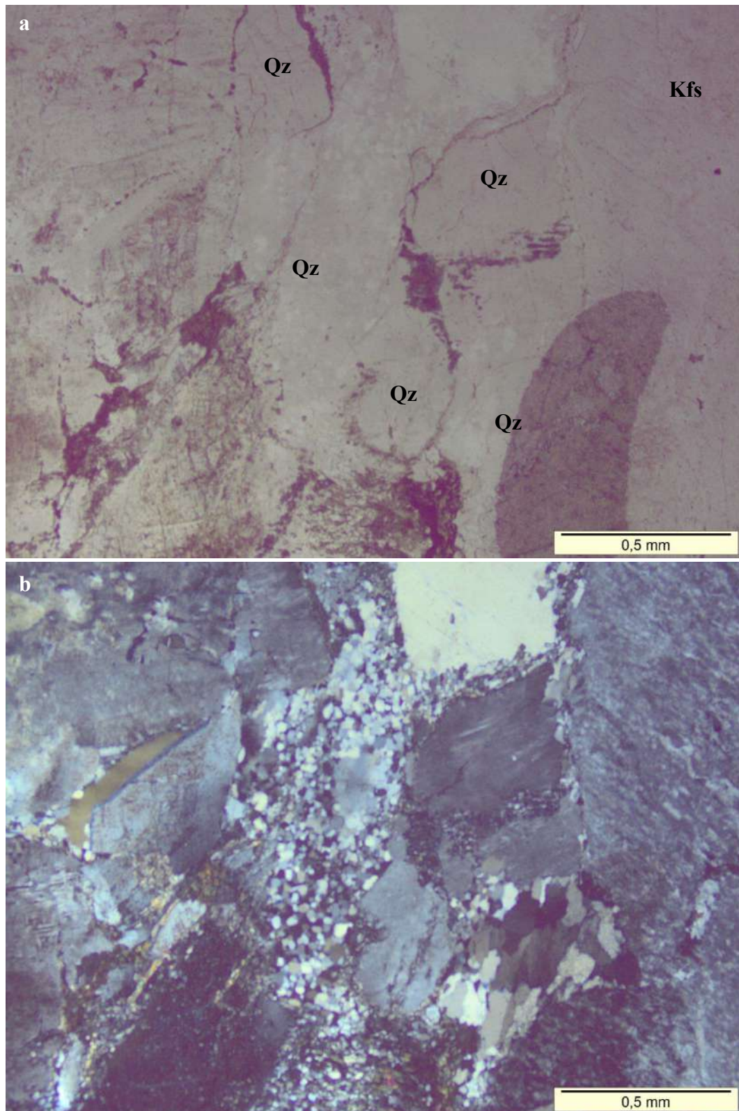
Figura 5.18 – Lâmina delgada da amostra SAC 7 mostrando diferentes gerações do quartzo, com e sem recuperação cristalina: a) nicóis paralelos; b) nicóis cruzados.
