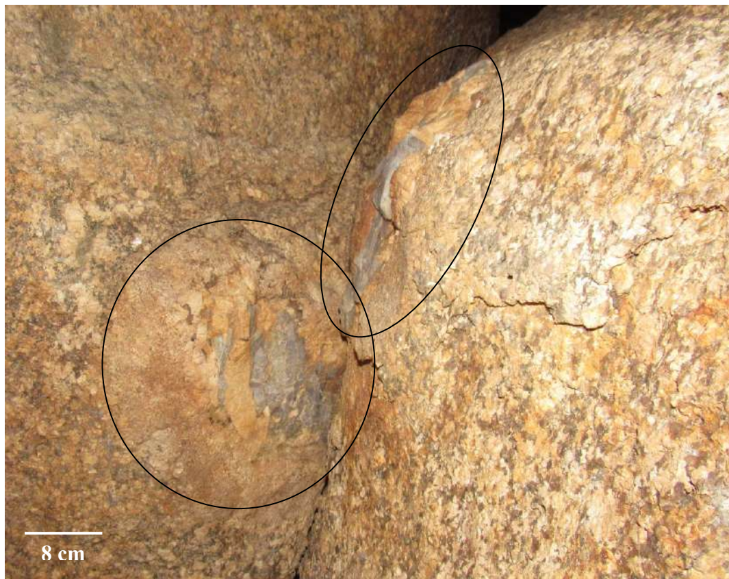
Figura 5.35 – Veio (ou bolsão) pegmatítico antes contínuo dividido em dois matacões distintos, mas ainda encostados um no outro.
